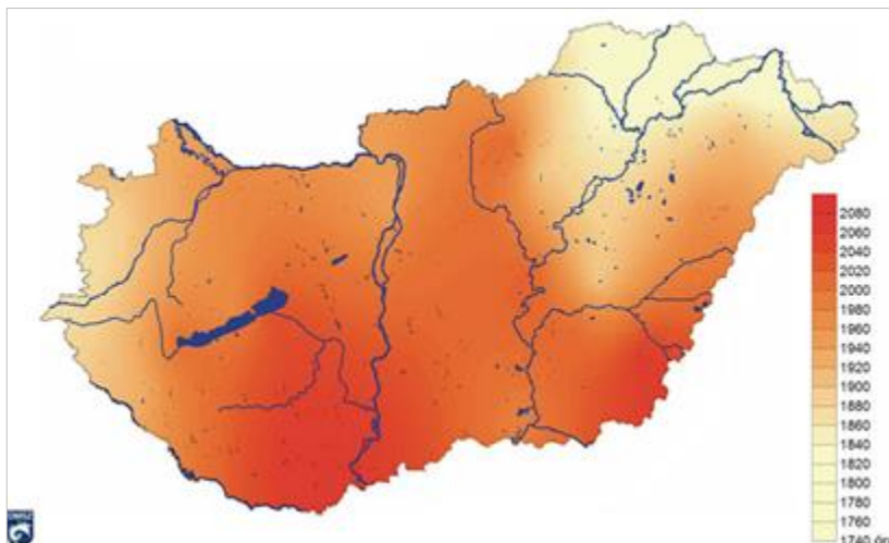
39. ábra Az évi átlagos napfénytartam (óra) Magyarországon az 1971-2000 közötti időszak alapján
