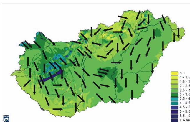
38. ábra Az évi átlagos szélességek [m/s] és az uralkodó szélirányok Magyarországon (2000-2009)
