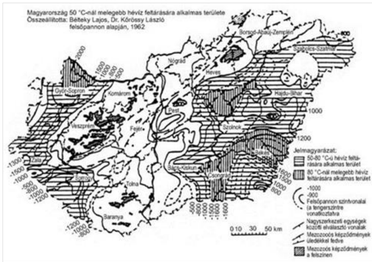
41. ábra Geotermikus energia - Magyarország 50 °C-nál melegebb hévíz feltárásának területei
